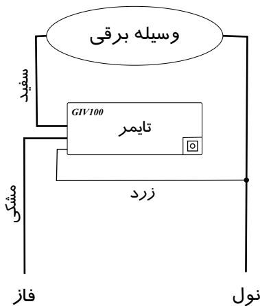
نقشه سیم کشی تایمر هوشمند گیو
